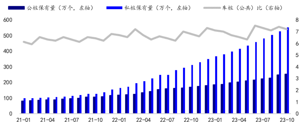
图2 中国充电桩保有量及车桩比
